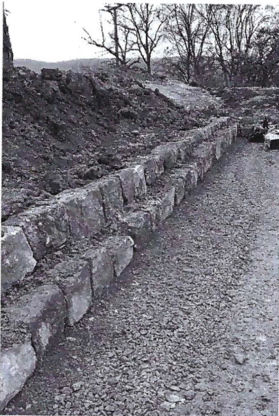
Die Bruchsteineinfassung passt sich optisch den örtlichen Gegebenheiten an und begrenzt den Parkplatz.
